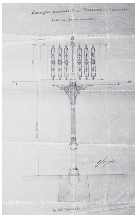
Nacrt željeznog stupa i ograde za Ljubićevu vilu iz 1876., izrađen od strane poduzeća Metlikovitz iz Trsta. Ovaj nacrt odgovara izvedenom stanju.
