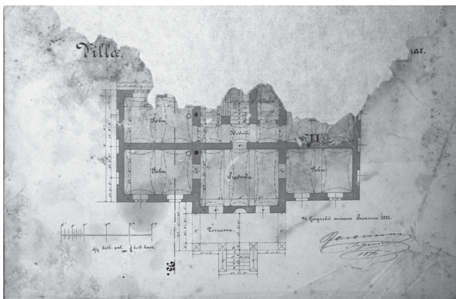
Nacrt pročelja arhitekta S. Jacominija za starigradsku vilu don Šime Ljubića iz 1872. godine (gore), i pripadajući tlocrt visokog prizemlja (dolje).
